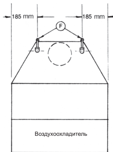
Вид спереди
