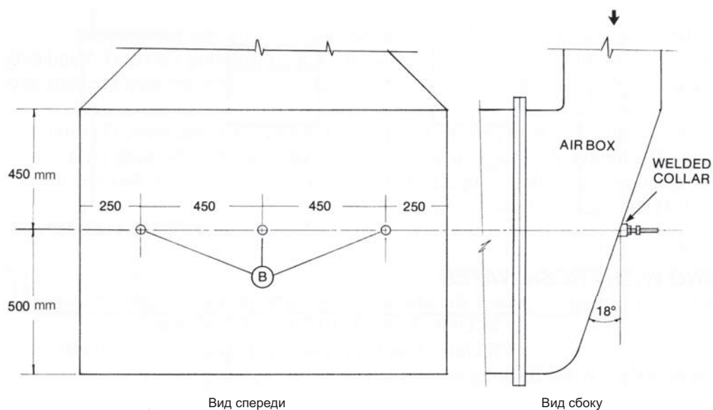
Вид спереди
